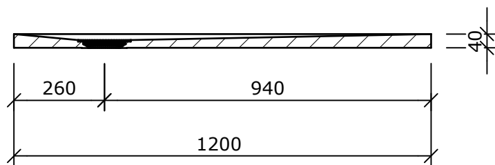
section A-A (1 : 15)
